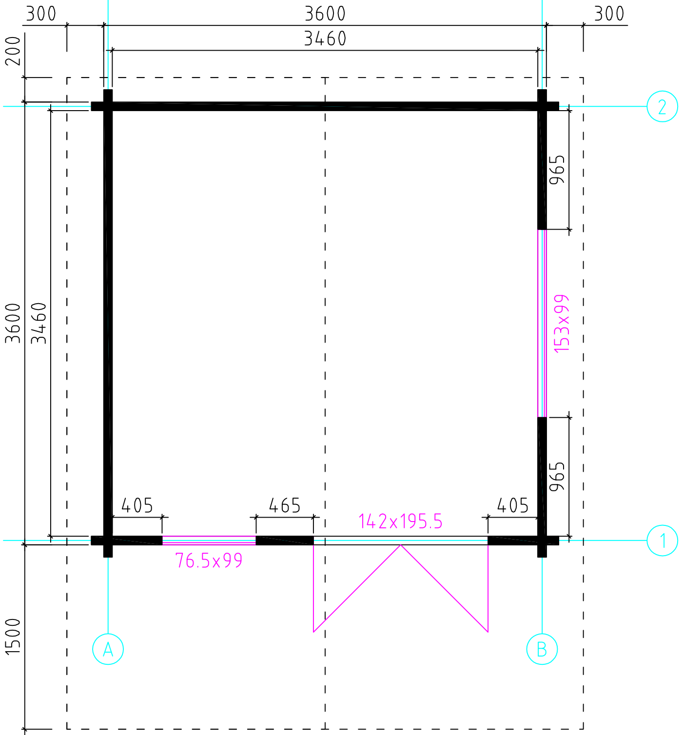
Grundplan
